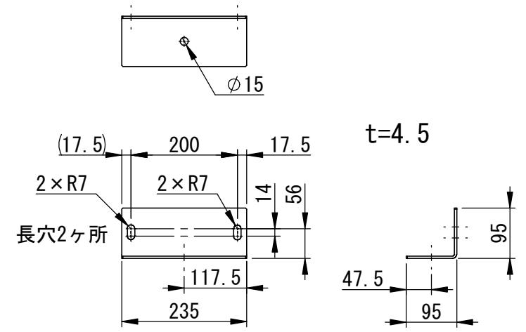
アンカーステー詳細図
