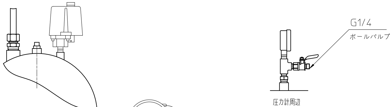
A 矢視図
