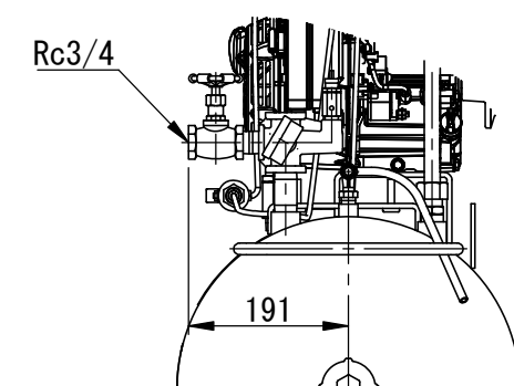
A 矢視図
