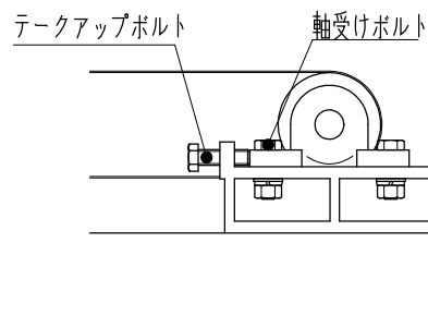
テークアップボルト部
