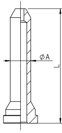
太口ノズル
