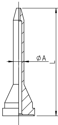
標準ノズル
