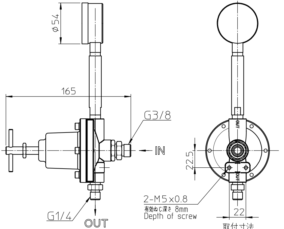
取付寸法 Mounting dimensions
